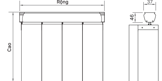
BẢN VẼ KỸ THUẬT
