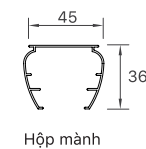
MẶT CẮT BIÊN DẠNG NHÔM
